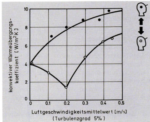
Bild 3: Konvektiver Wärmeübergangskoeffizient an der Stirn eines auf 34 °C beheizten künstlichen Kopfes bei aufwärts und abwärts gerichteter Luftströmung mit geringer Turbulenz, in Abhängigkeit von der Luftgeschwindigkeit, bei einer Umgebungstemperatur von 23 °C.
