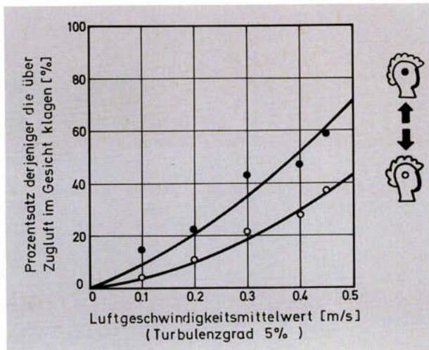
Bild 1: Prozentsatz der Menschen, die über Zugluft im Gesicht klagen bei aufwärts und abwärts gerichteter Luftströmung mit geringer Turbulenz, in Abhängigkeit von der Luftgeschwindigkeit, bei einer Umgebungstemperatur von 23 °C.
