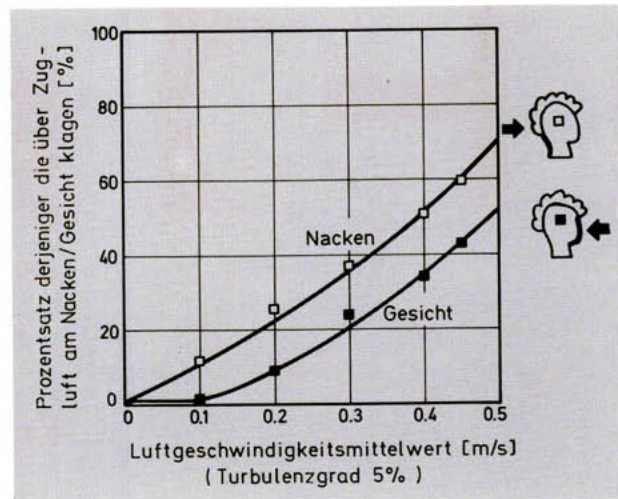
Bild 2: Prozentsatz der Menschen, die über Zugluft im Gesicht und im Nacken klagen bei horizontaler Luftströmung mit geringer Turbulenz von vorne und von hinten, in Abhängigkeit von der Luftgeschwindigkeit, bei einer Umgebungstemperatur von 23 °C.
