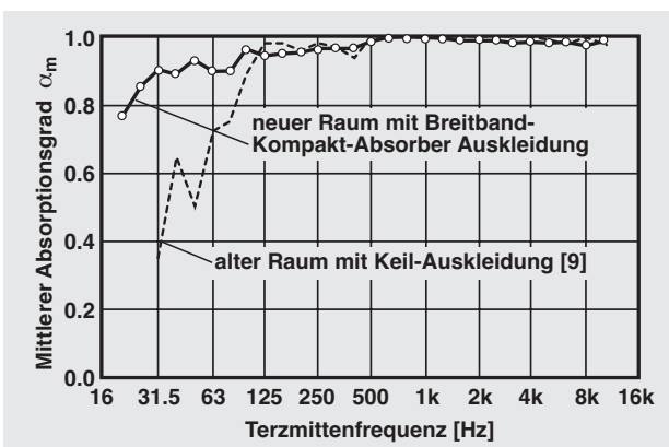
Bild 3: Mittlerer Absorptionsgrad der Raumauskleidung in Abhängigkeit von der Terzmittenfrequenz, ermittelt aus Messungen nach Diestel [8].
