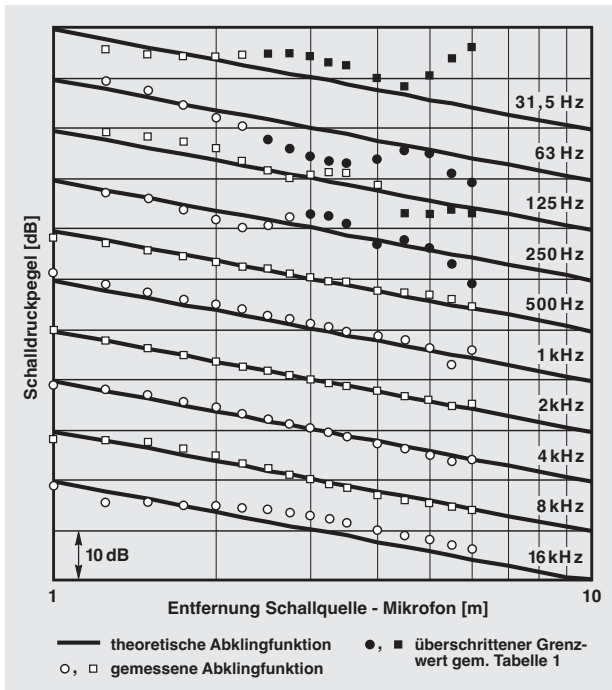
Bild 2: Gemessene und theoretische Abklingfunktion entlang einer radial von der Position der Schallquelle gezogenen Bahn für die Terzen bei den Oktavmittelfrequenzen von 31,5 Hz bis 16 kHz.
